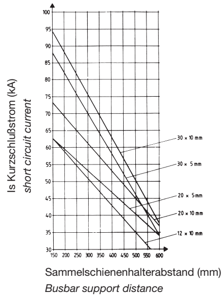
Kurzschlussfestigkeitsdiagramm (60 mm) Diagram of short circuit capability (60 mm)
