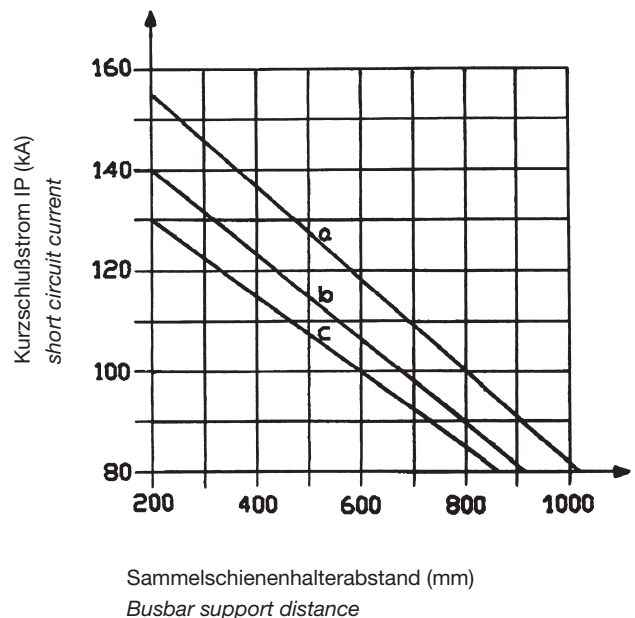
Kurzschlussfestigkeitsdiagramm (185 mm) Diagramm of short circuit capability (185 mm)
